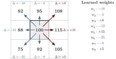
PIDINet (Su et al., 2021)
