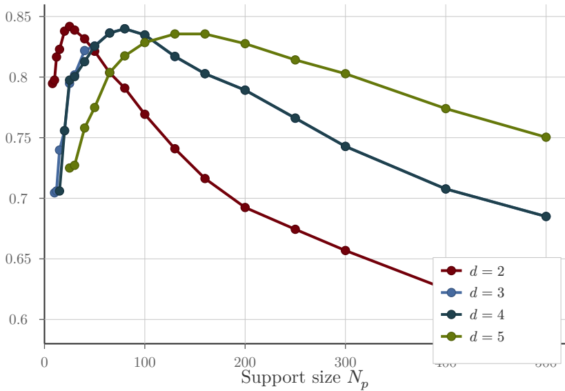
ODS F-score
