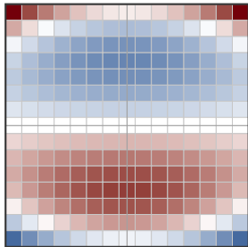
K_y^{\text{square}}
