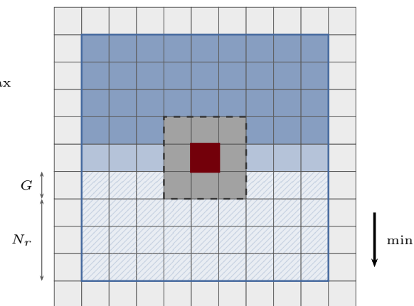
SO-CFAR
