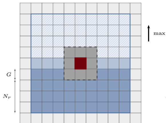
GO-CFAR
