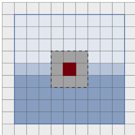
GO-CFAR
