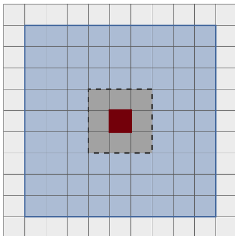
CA-CFAR
