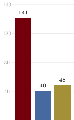
VRAM (GB)
