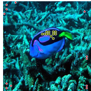
12 pos, 12 neg
