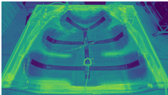
CIELAB L^*
