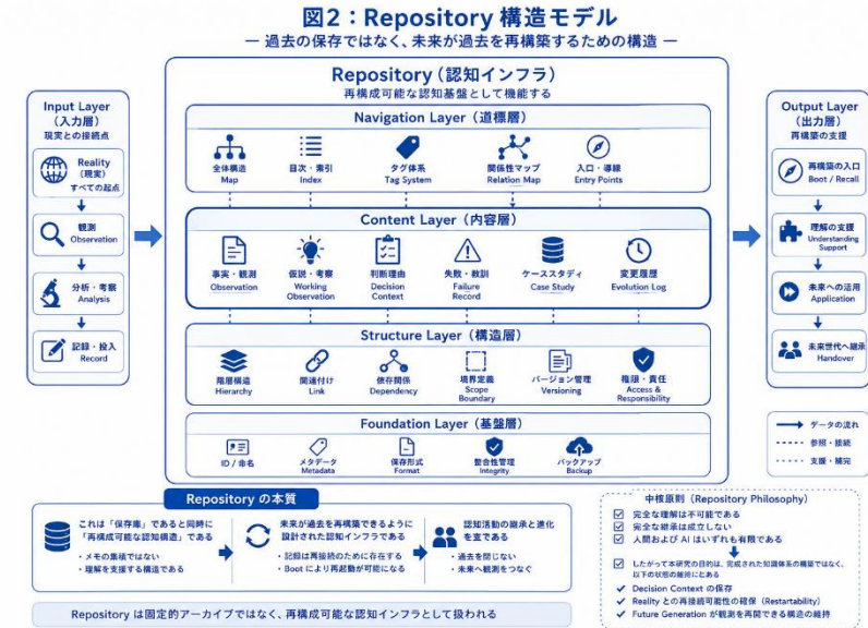
図 2 Repository構造モデル
