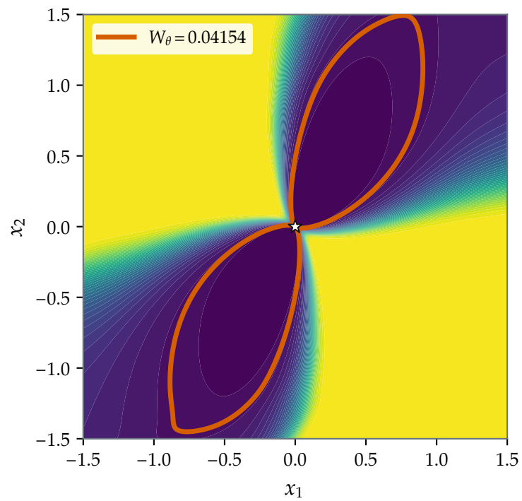
Example VI.2 (Cubic core) Verified sublevel set
