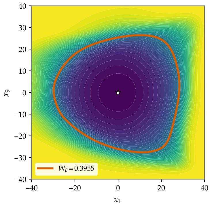
Example VI.3 (10D) Tested sublevel set
