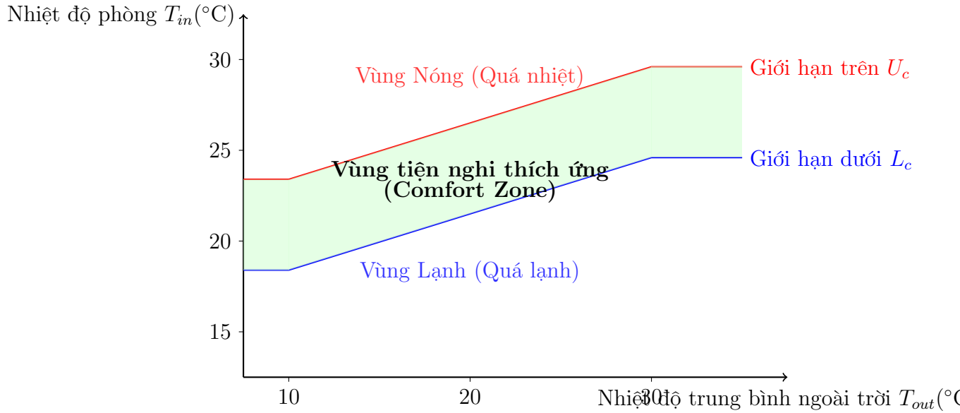
Hình 2: Dải giới hạn nhiệt độ tiện nghi thích ứng theo tiêu chuẩn ASHRAE Standard 55
