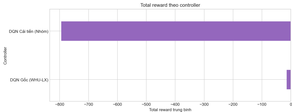
Hình 8: Tổng điểm thưởng (Reward) trung bình tích lũy thu được của hai bộ điều khiển DQN.
