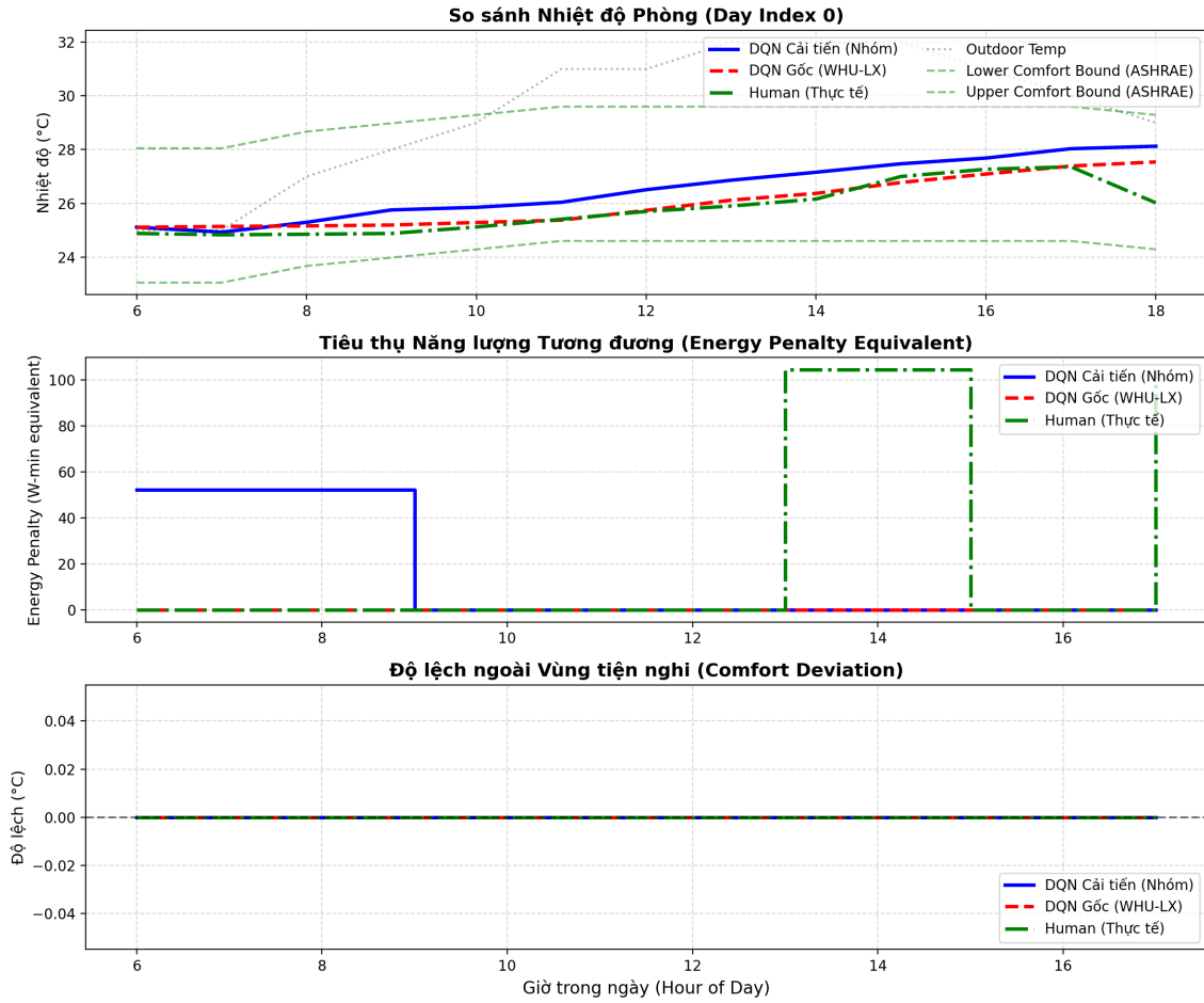
Hình 7: So sánh chuỗi thời gian vận hành chi tiết (Nhiệt độ phòng, Năng lượng tiêu thụ tương đương và Độ lệch tiện nghi) giữa ba bộ điều khiển trên ngày thử nghiệm tiêu biểu (Day 0).
