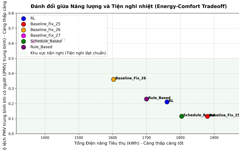
Hình 4: Quan hệ đánh đổi giữa điện năng tiêu thụ và chất lượng tiện nghi nhiệt của các bộ điều khiển.
