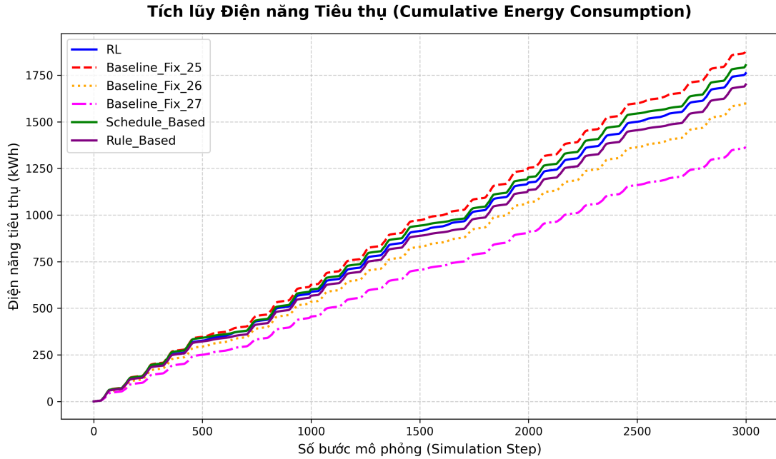
Hình 3: So sánh điện năng tích lũy của DQN với các chiến lược điều khiển nền trong kịch bản mùa nóng Thành phố Hồ Chí Minh.
