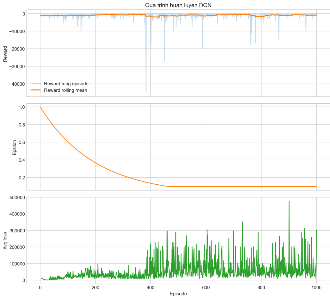
Hình 5: Tiến trình huấn luyện tác tử DQN cải tiến trên môi trường surrogate XGBoost (Reward, Epsilon và Average Loss theo số episode).
