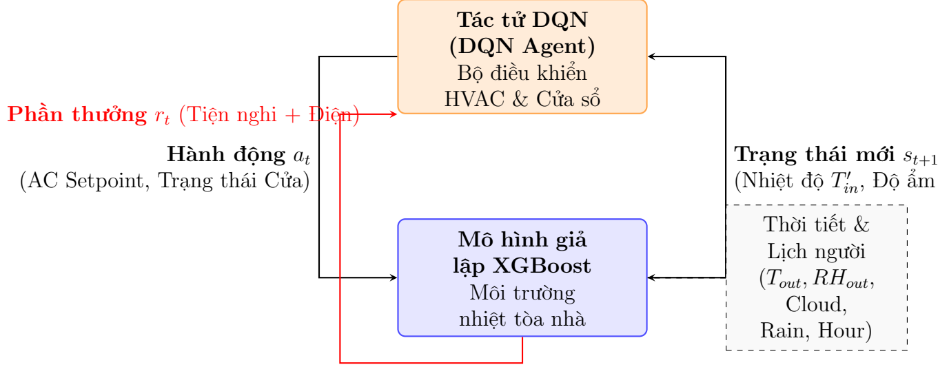
Hình 1: Sơ đồ khối hệ thống lai điều khiển HVAC phối hợp cửa sổ XGB-DQN
