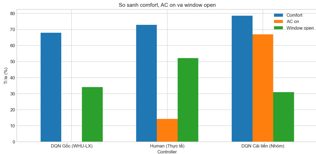
Hình 6: So sánh tỷ lệ thời gian tiện nghi nhiệt (Comfort), bật điều hòa (AC on) và mở cửa sổ (Window open) của ba bộ điều khiển.
