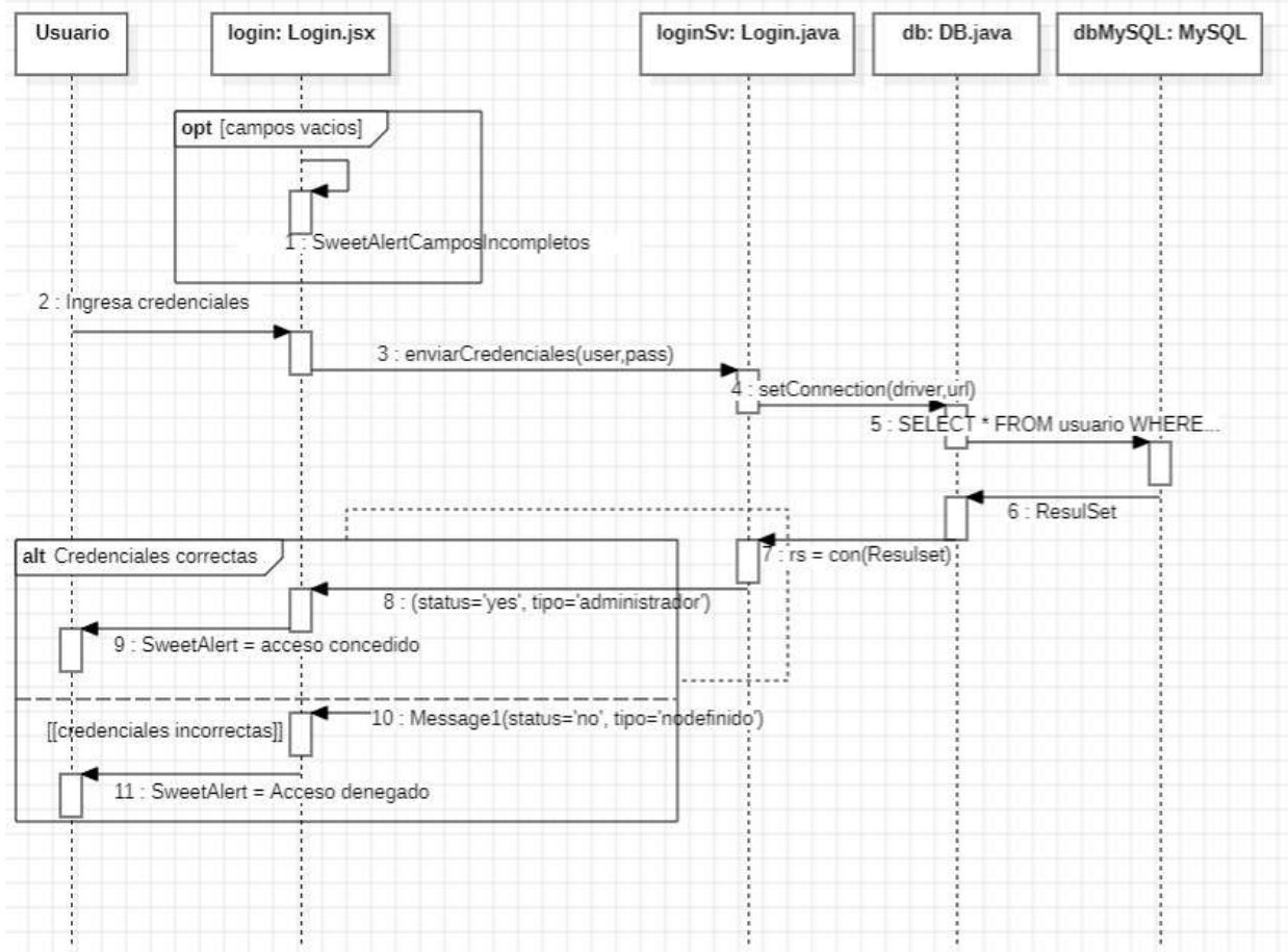
Figura 4. Diagrama de Secuencia — Inicio de Sesión
