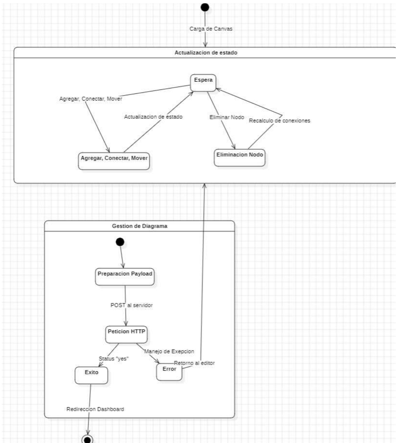
Figura 7. Diagrama de Estados — Backend
