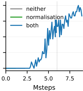
pick-place
