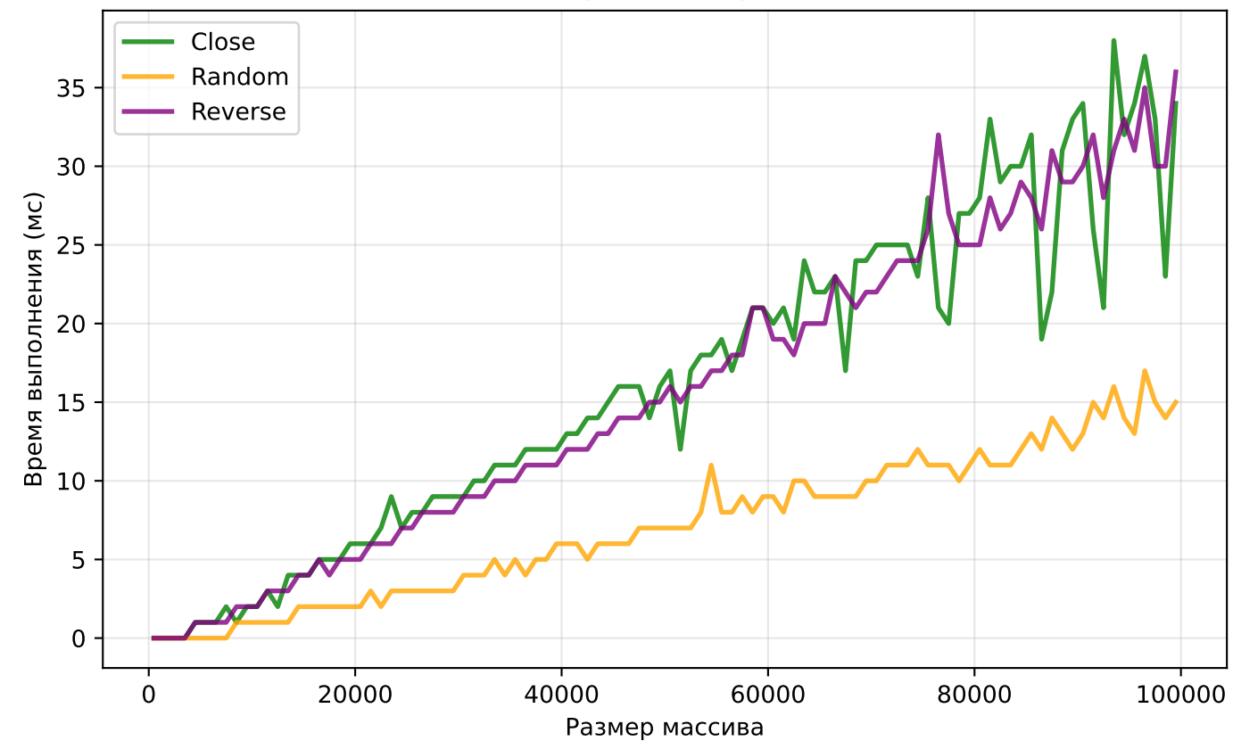
Сравнение типов массивов (IntroSort)
