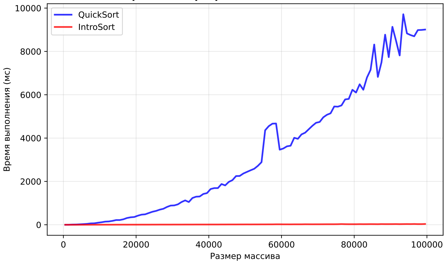
Обратно отсортированный массив (Reverse)
