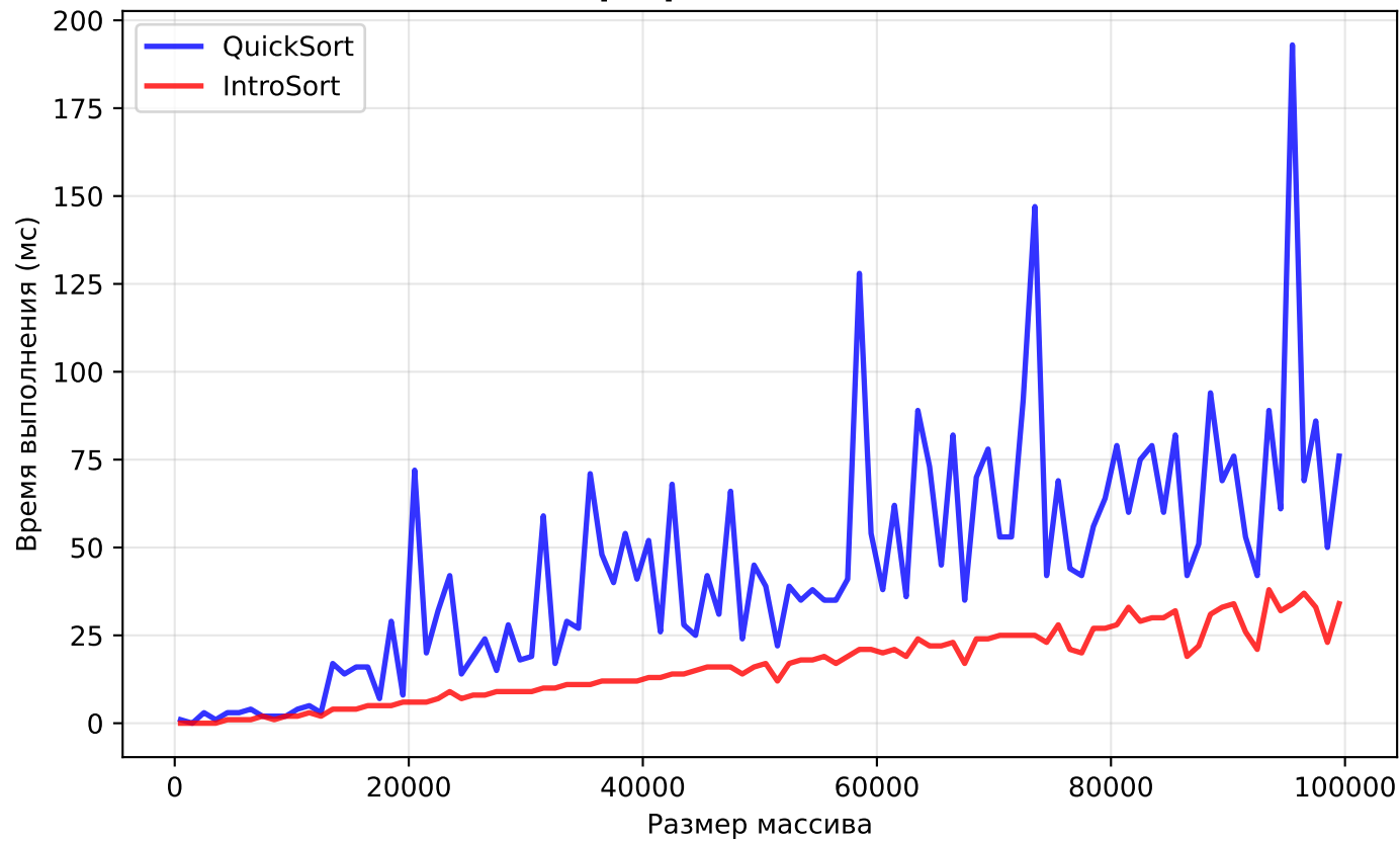
Почти отсортированный массив (Close)
