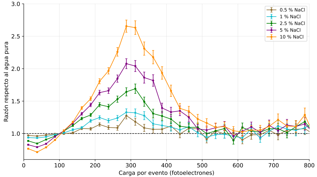
Figura 4: Razón entre la distribución normalizada de cada medio con NaCl y la del agua pura, en intervalos de 25 pe y sin suavizar, con error de Poisson.
