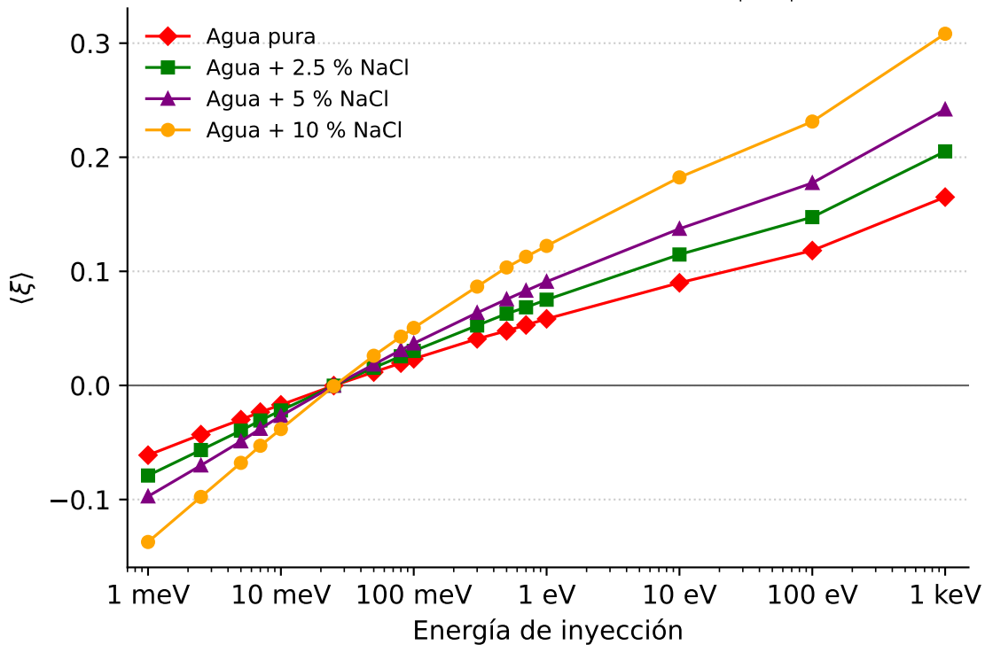
Definición de la tesis: \xi por colisión, \langle \ln(E_{\text{pre}}/E_{\text{post}}) \rangle
