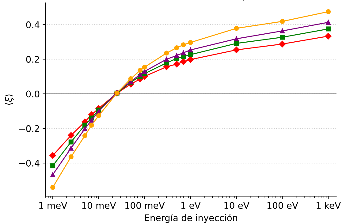
Definición inicial (reemplazada): \langle \ln(E_0/E_{\text{cap}})/N \rangle por historia
