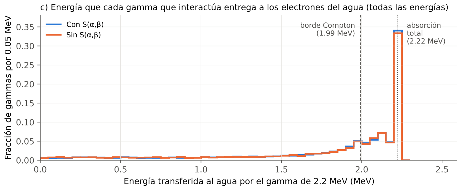
Gammas de 2.223 MeV de la captura en hidrógeno. b): intervalos de 1 cm con al menos 50 gammas. c): suma de las pérdidas del gamma primario en sus interacciones Compton, fotoeléctrica y de pares.
