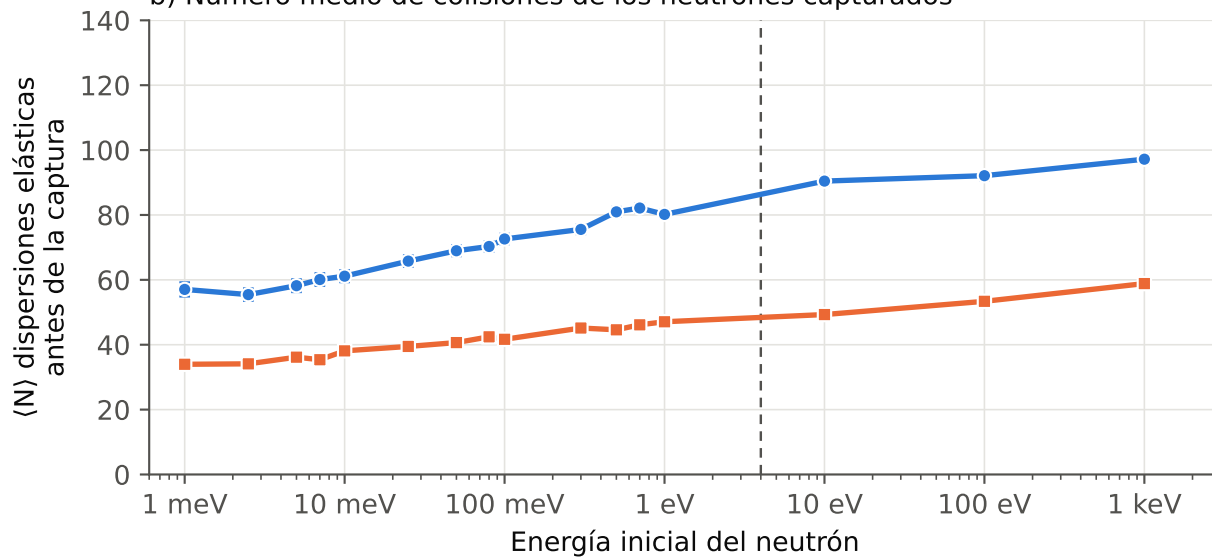
b) Número medio de colisiones de los neutrones capturados
