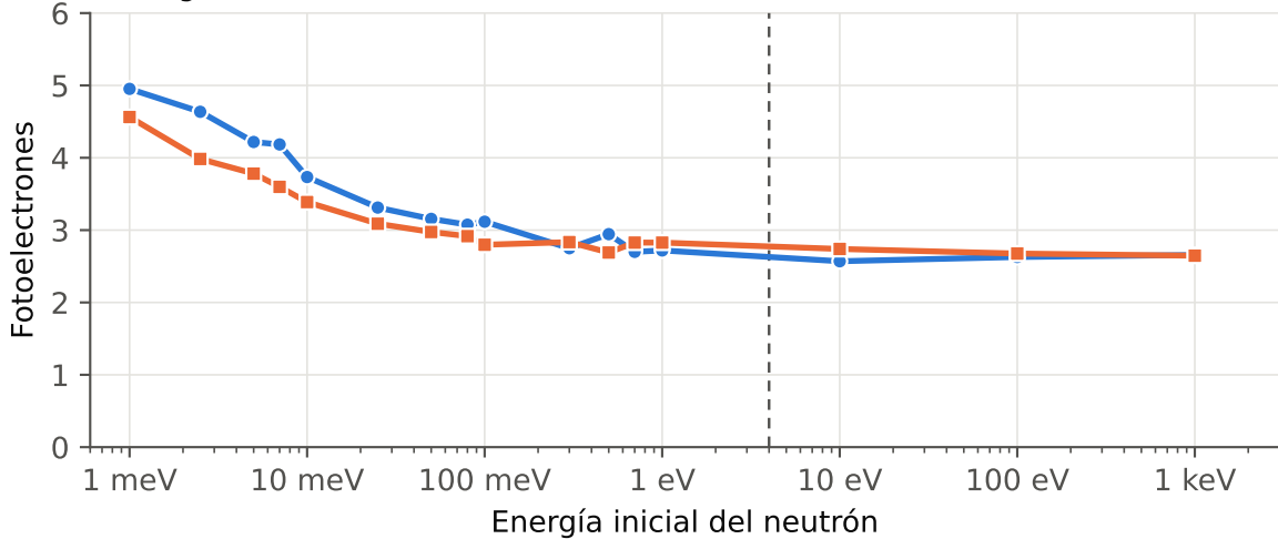
c) Carga media de los eventos con señal
