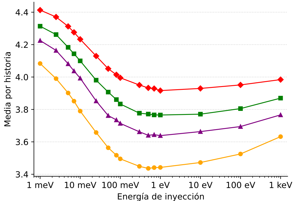
Pasos Transportation por neutrón incidente
