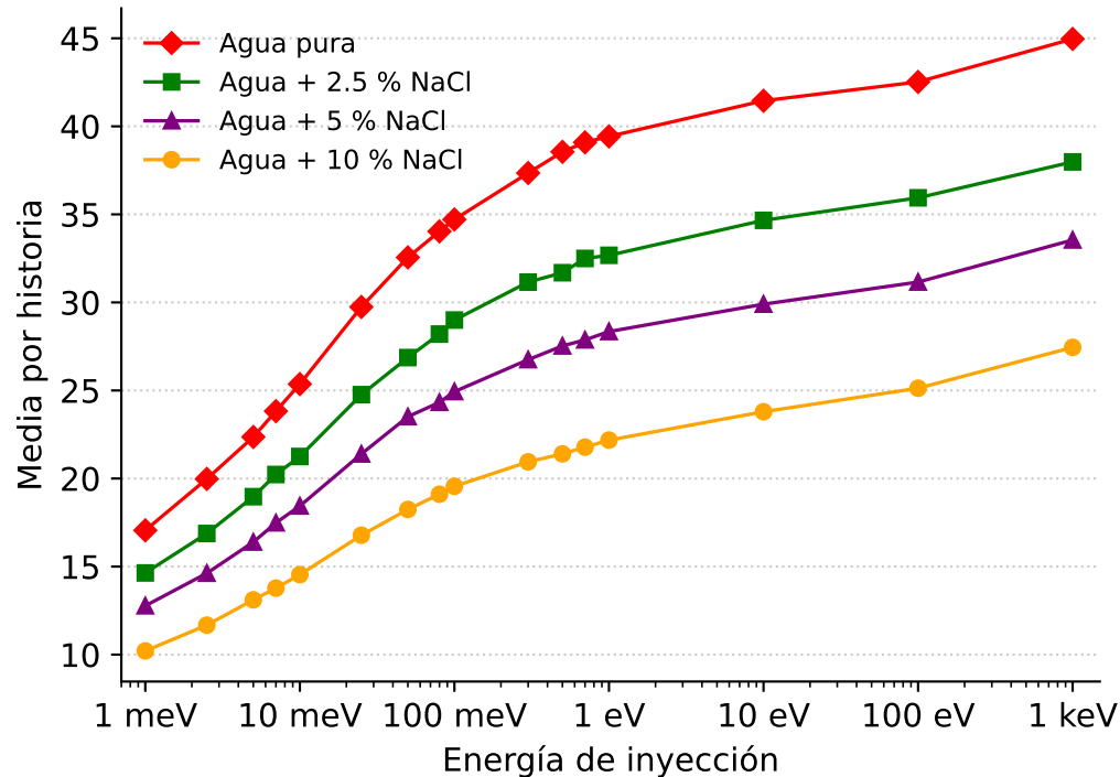
Pasos hadElastic por neutrón incidente
