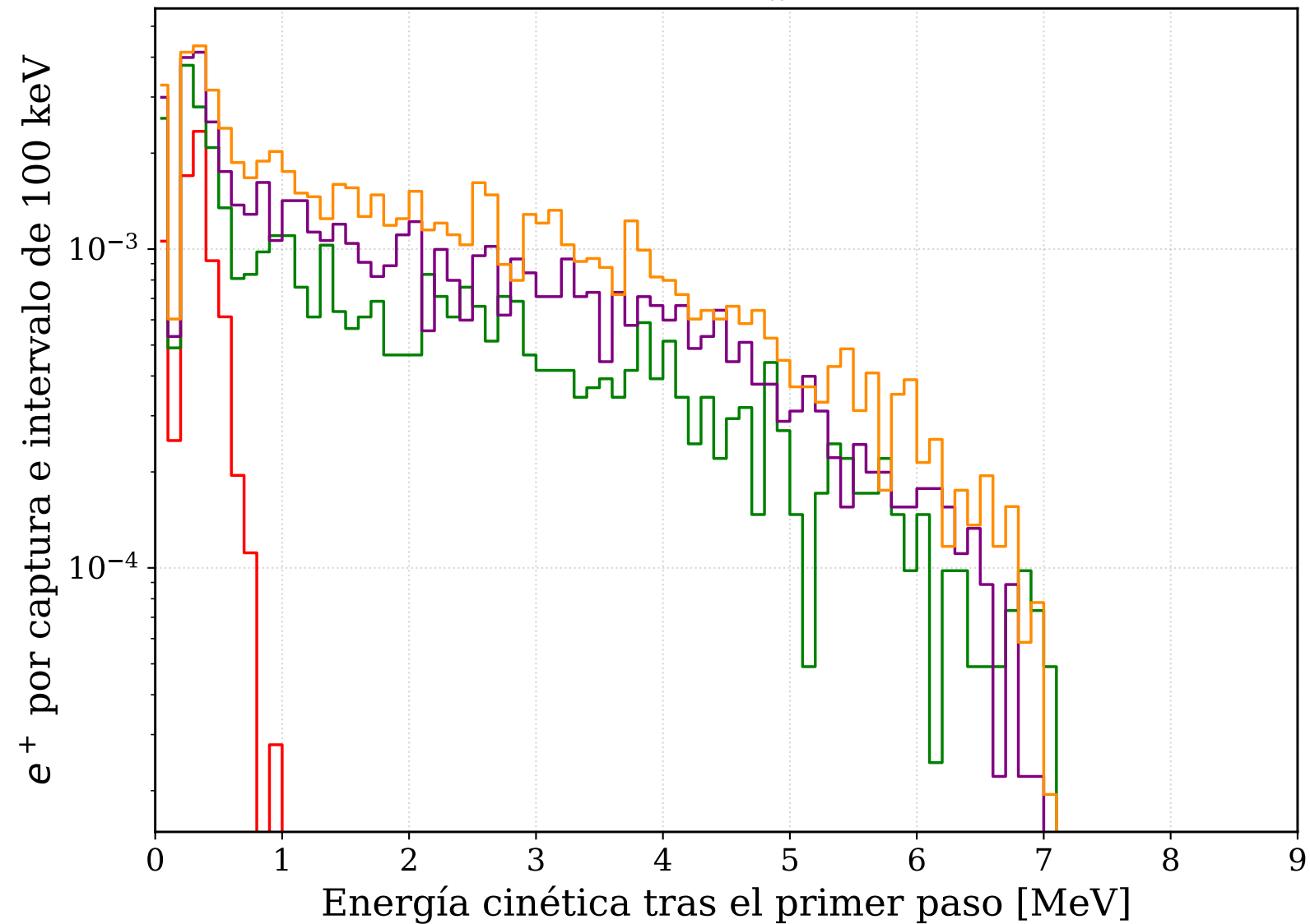
Positrones, E_n = 1 eV
