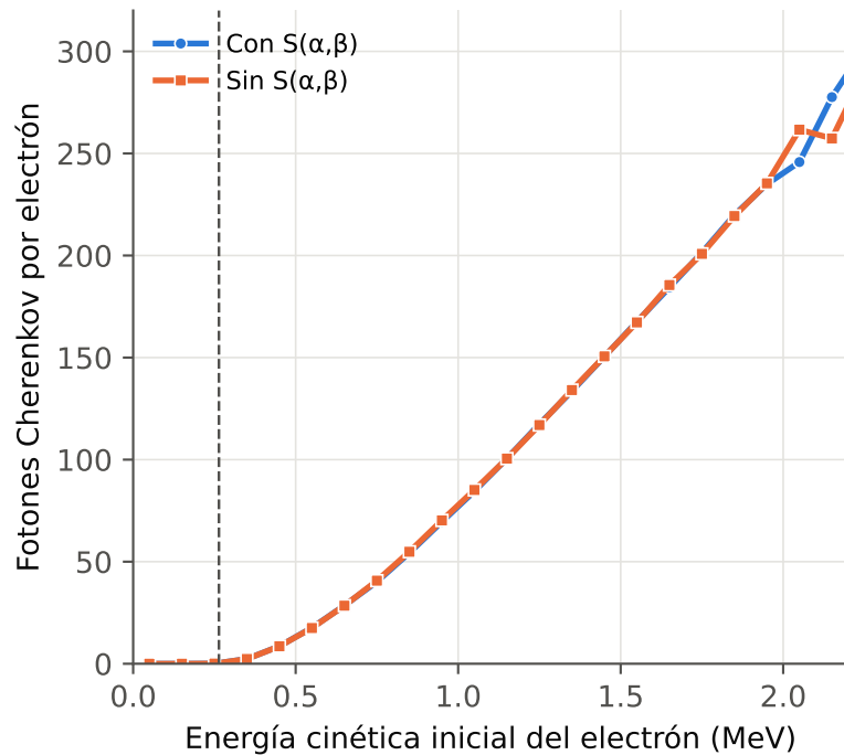
b) Luz emitida según la energía del electrón
