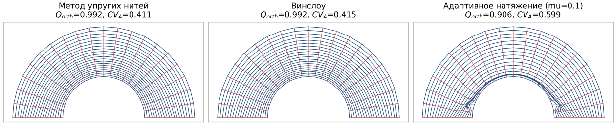
Рис. 3: Сетки полукольца. Метод упругих нитей показан после теоретически предусмотренной балансировки жёсткостей.
