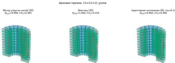
Рис. 7: Сетки арковой призмы 11^3 : упругие нити после балансировки, Винслоу и адаптивное натяжение.
