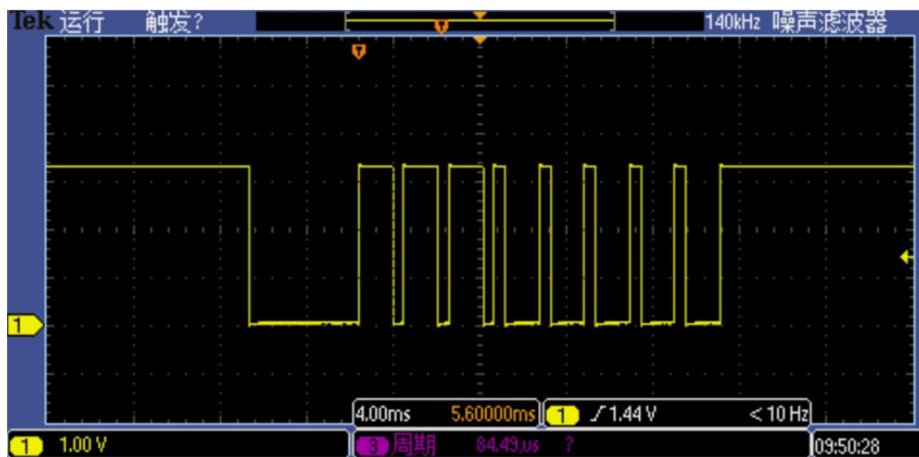
0X07 地址时序图
