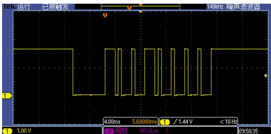
0X09 地址时序图
