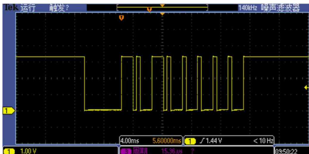
0X05 地址时序图
