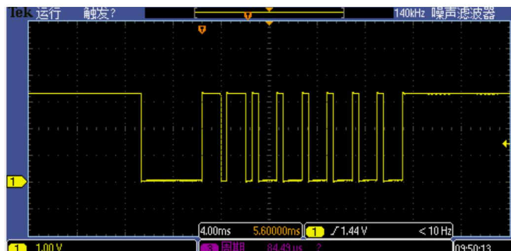
0X03 地址时序图
