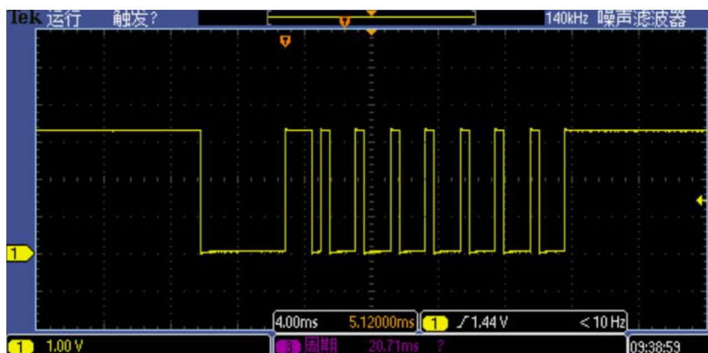
0X01 地址时序图
