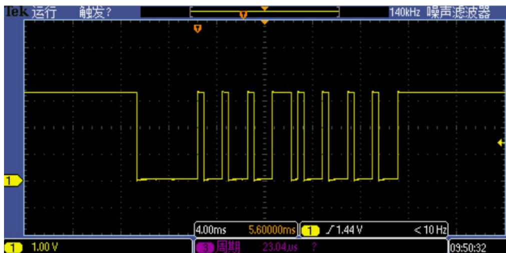
0X08 地址时序图
