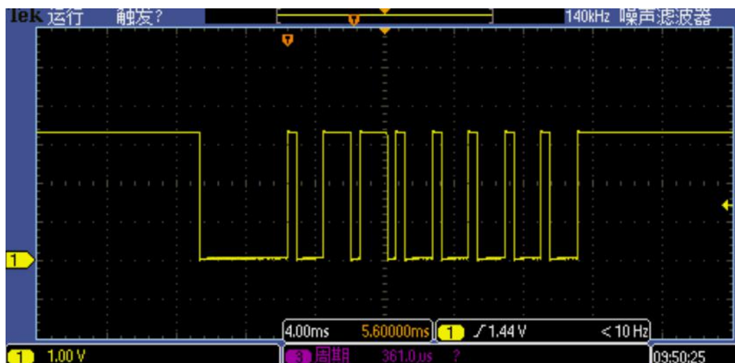
0X06 地址时序图
