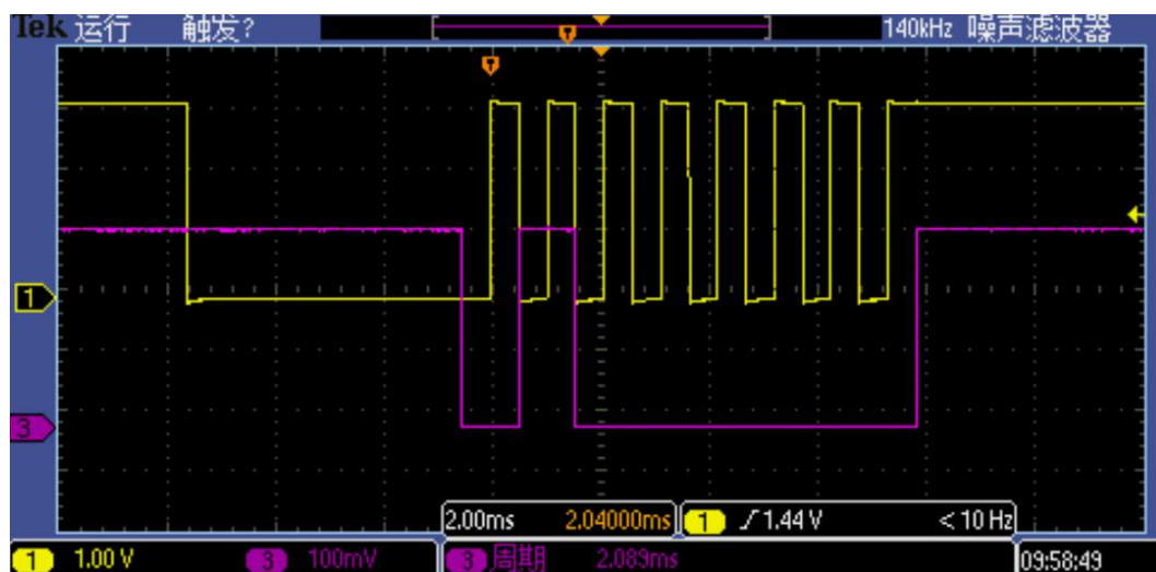
0X02 地址时序图
