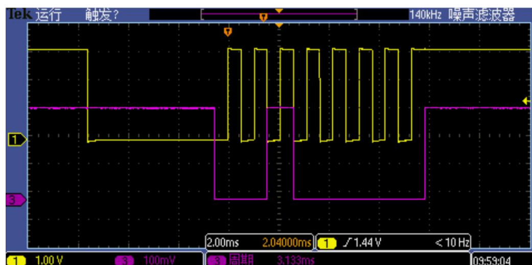
0X04 地址时序图
