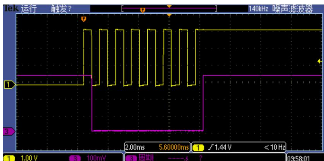
0X01 地址时序图
