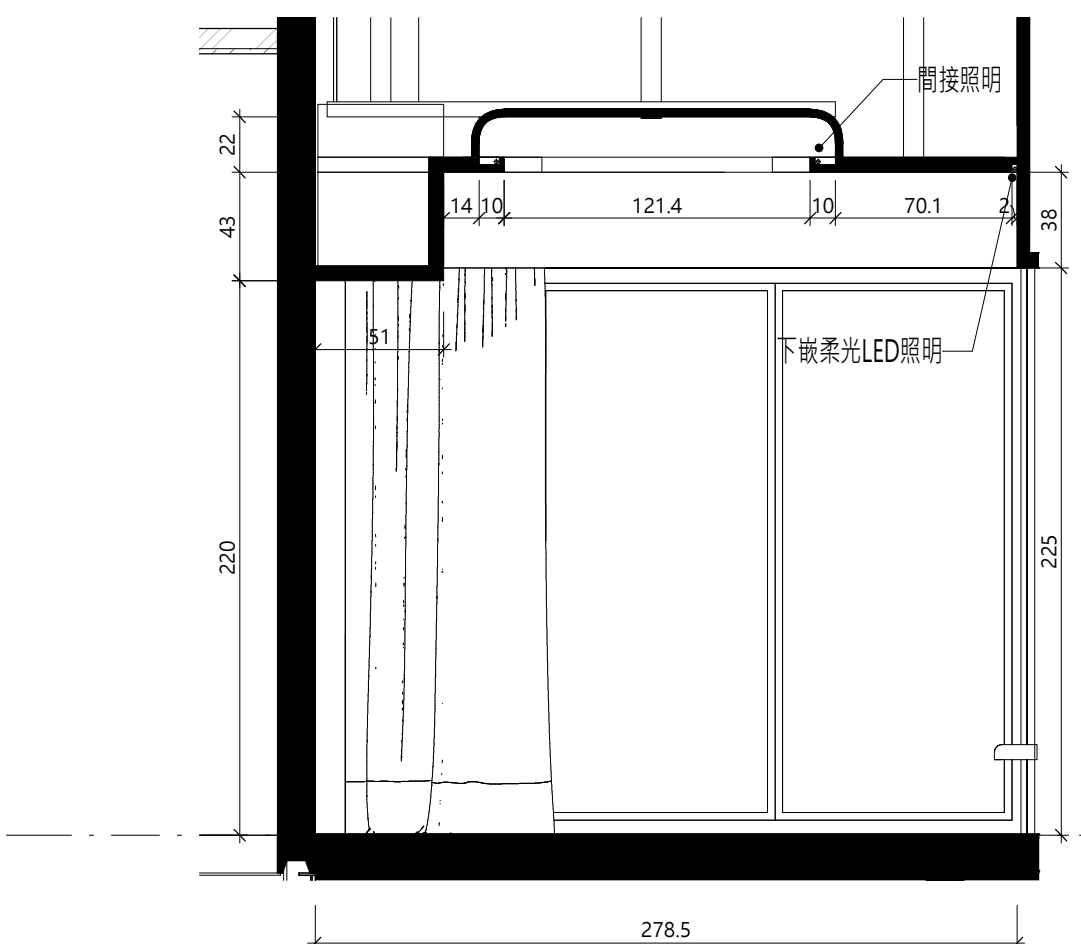
3 天花詳圖 A1=NTS A3=NTS
