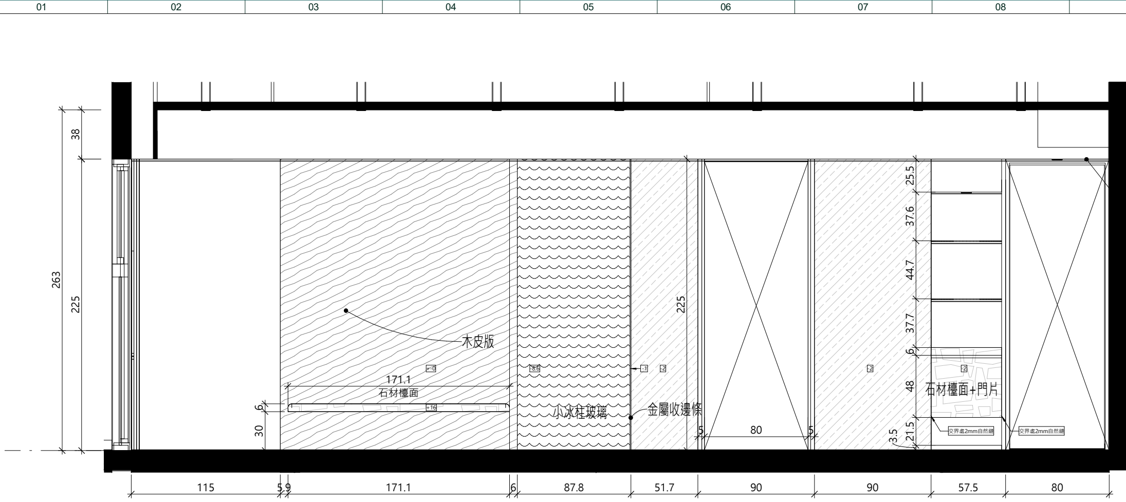
2 櫃體圖2 A1=NTS A3=NTS
