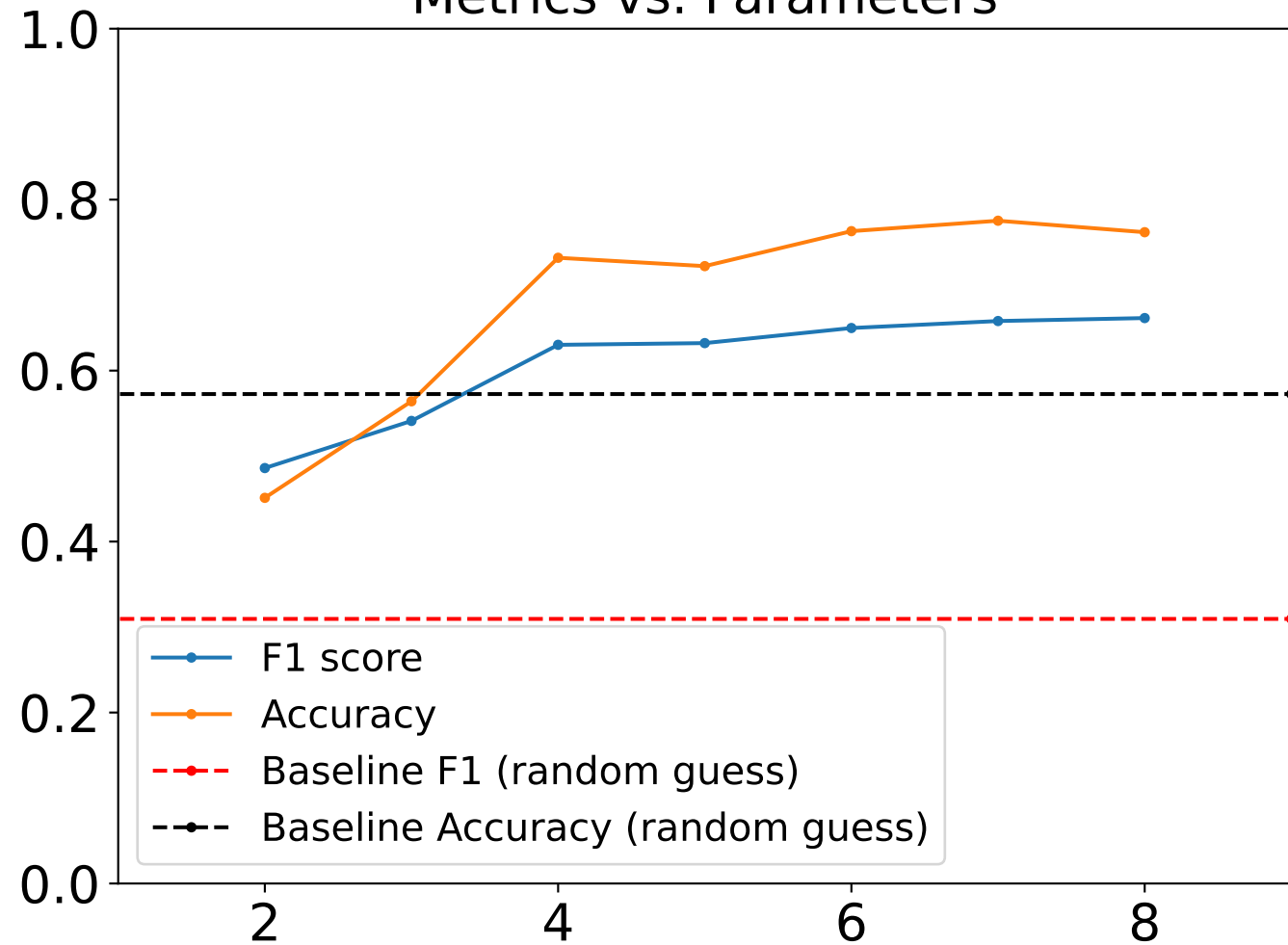
Metrics vs. Parameters
