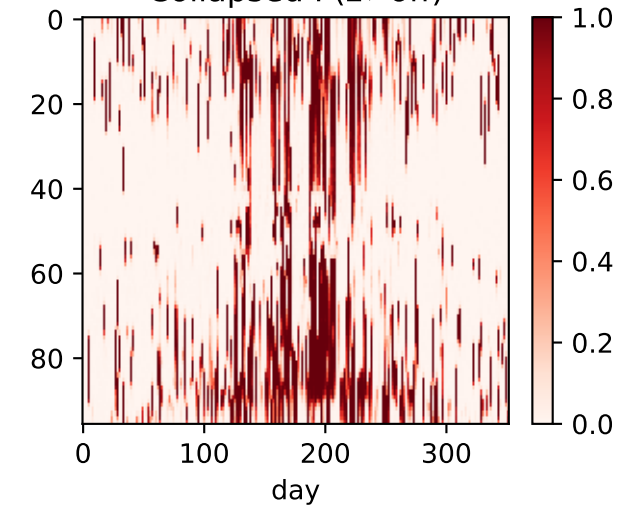
Collapsed P(z \neq \text{off})
