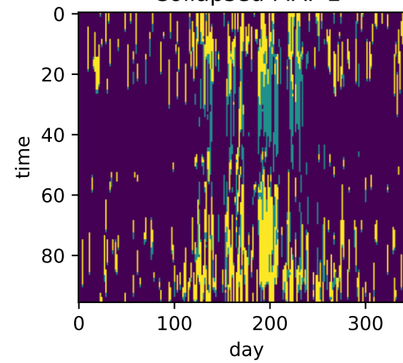
Collapsed MAP z
