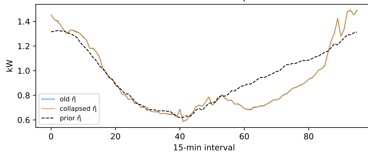
Posterior mean \eta
