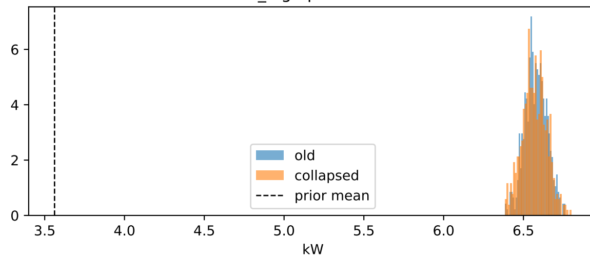
\Theta_{\text{high}} posterior
