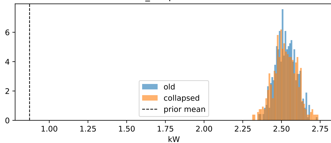
\Theta_{\text{low}} posterior
