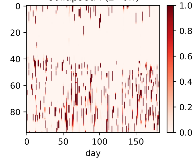
Collapsed P(z \neq \text{off})
