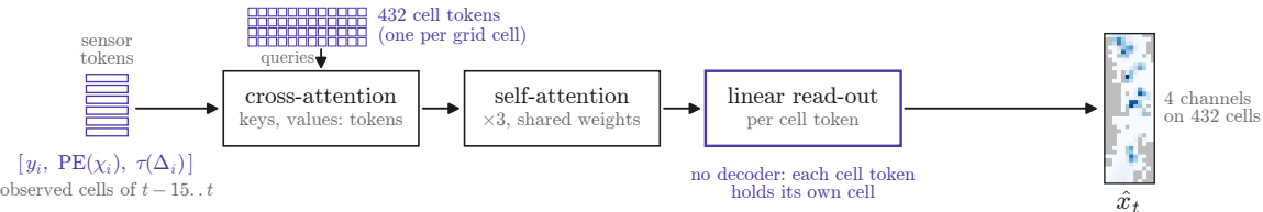
(b) Senseiver-G (ours)
