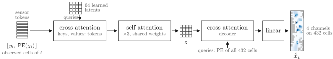
(b) Senseiver-G (ours)
