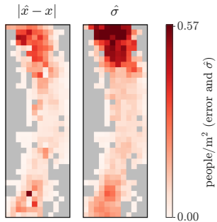
EnKF
