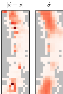
DINCAE
