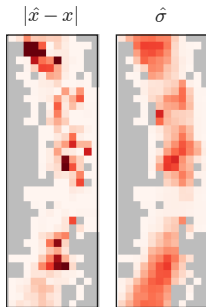
DINCAE
