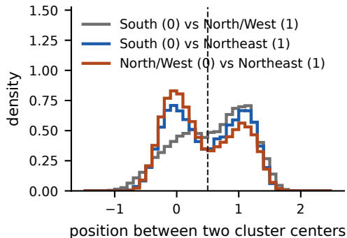
(d) Pairs of clusters
