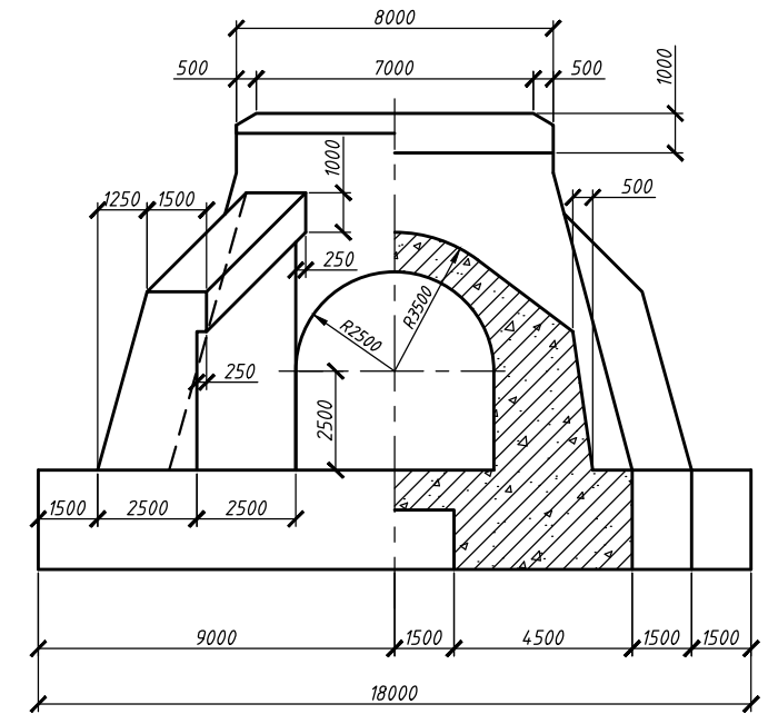
2-2剖面图
