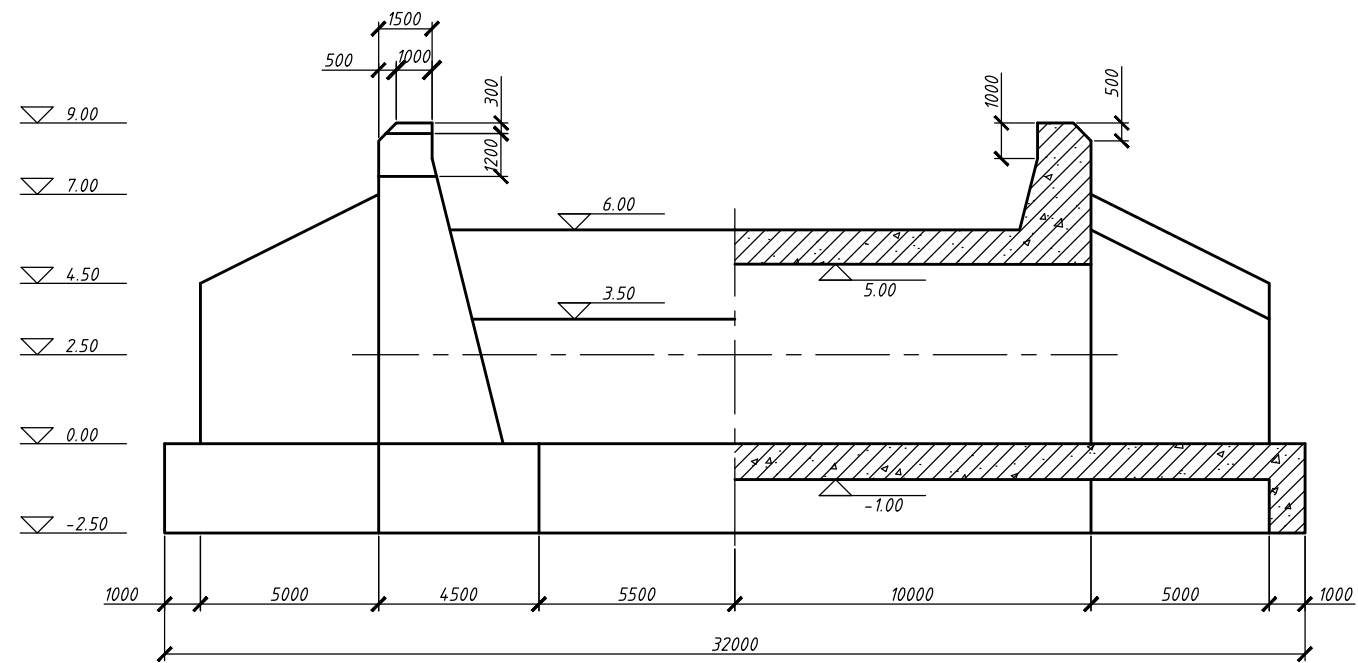
1-1剖面图
