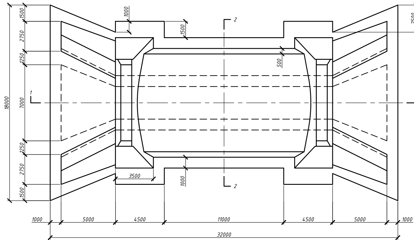
平面图
