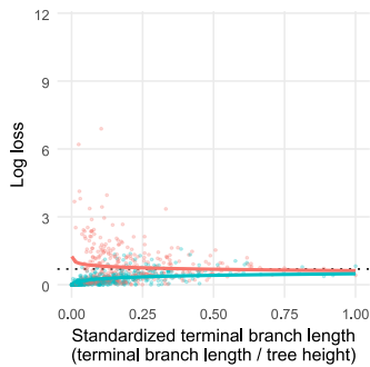
Q_4
