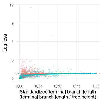
Q_9
