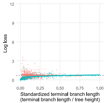
Q_5
