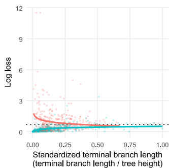
Q_{10}
