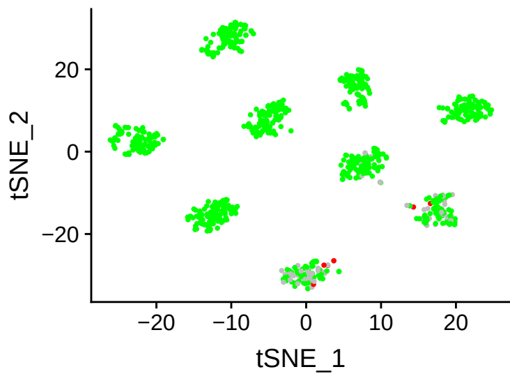
ENSG00000135549
