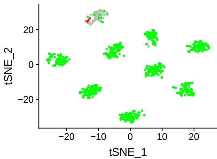
ENSG00000164265
