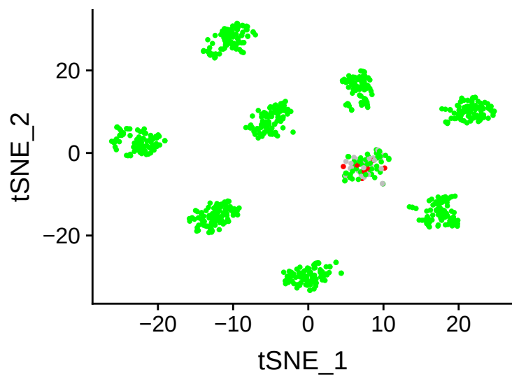
ENSG00000154556
