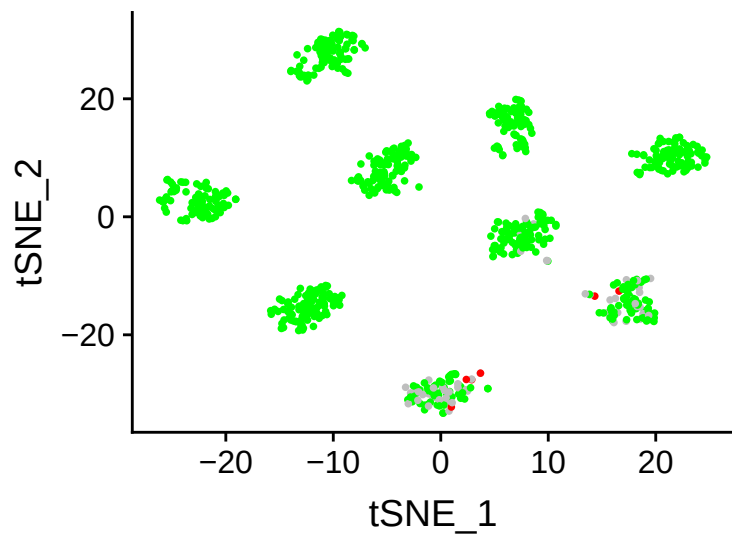
ENSG00000131969
