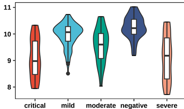
HLA-DRA
