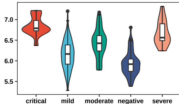
TFPI
