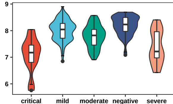
G6PD
