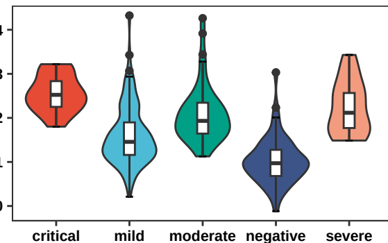
GSR
