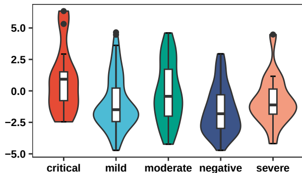
F12
