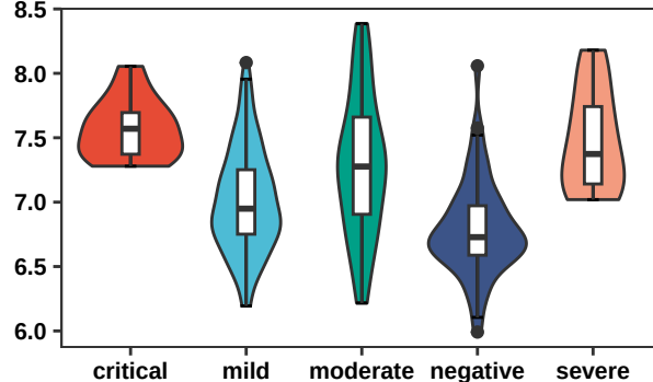
HLA-DRA
