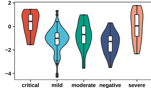
TFPI
