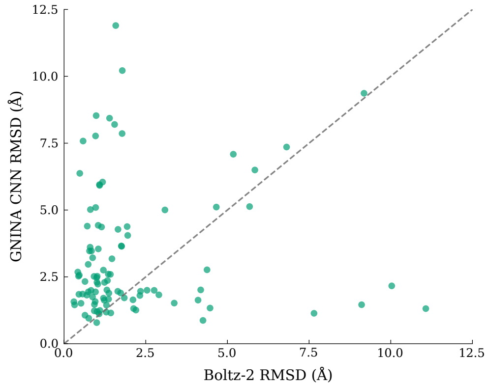
Boltz-2 vs GNINA CNN
