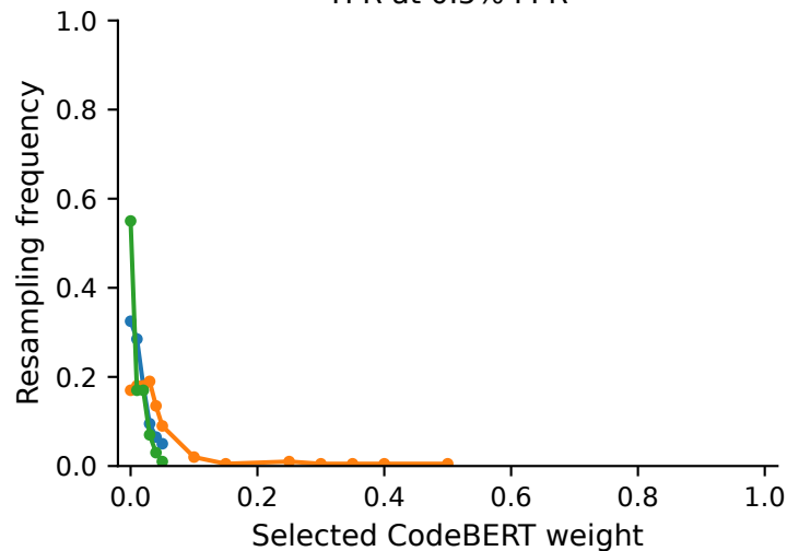
TPR at 0.5% FPR
