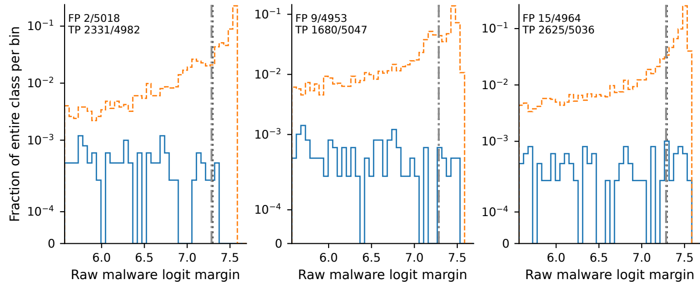
Win32
