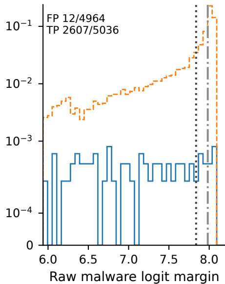
.NET
