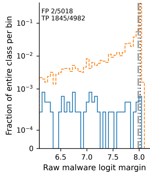
Win32
