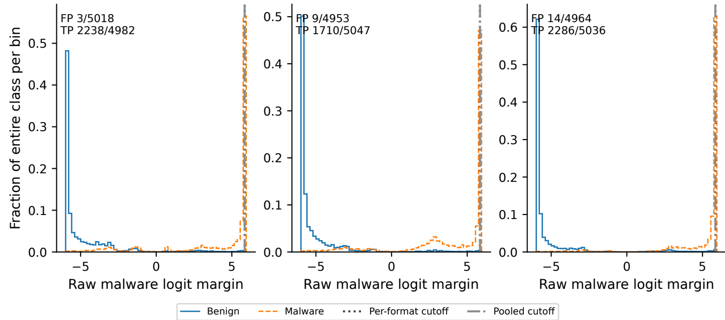
Win32
