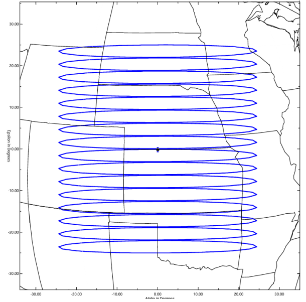
图 1: OneWeb Ku-band 16-beam 在 (\alpha, \epsilon) 天線平面上的 footprint；每個輪廓代表一個 spot beam 的覆蓋區。
