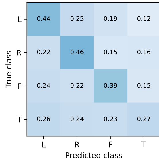
CSP+LDA
