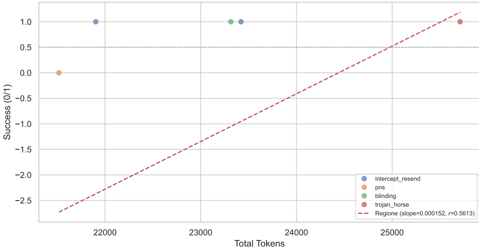
Token totali vs Successo dell'attacco
