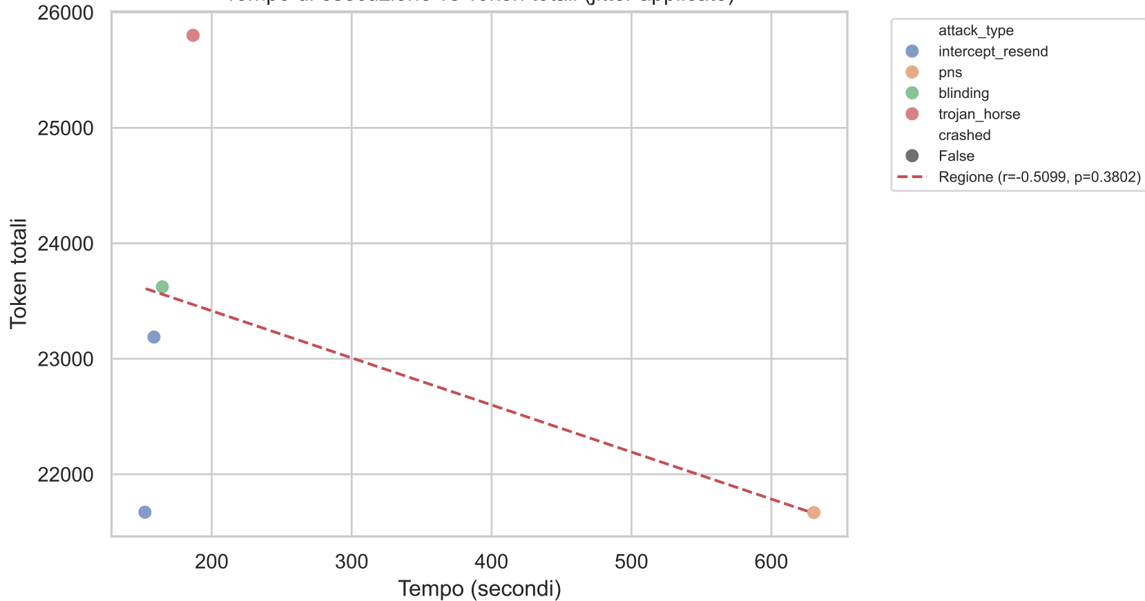
Tempo di esecuzione vs Token totali (jitter applicato)
