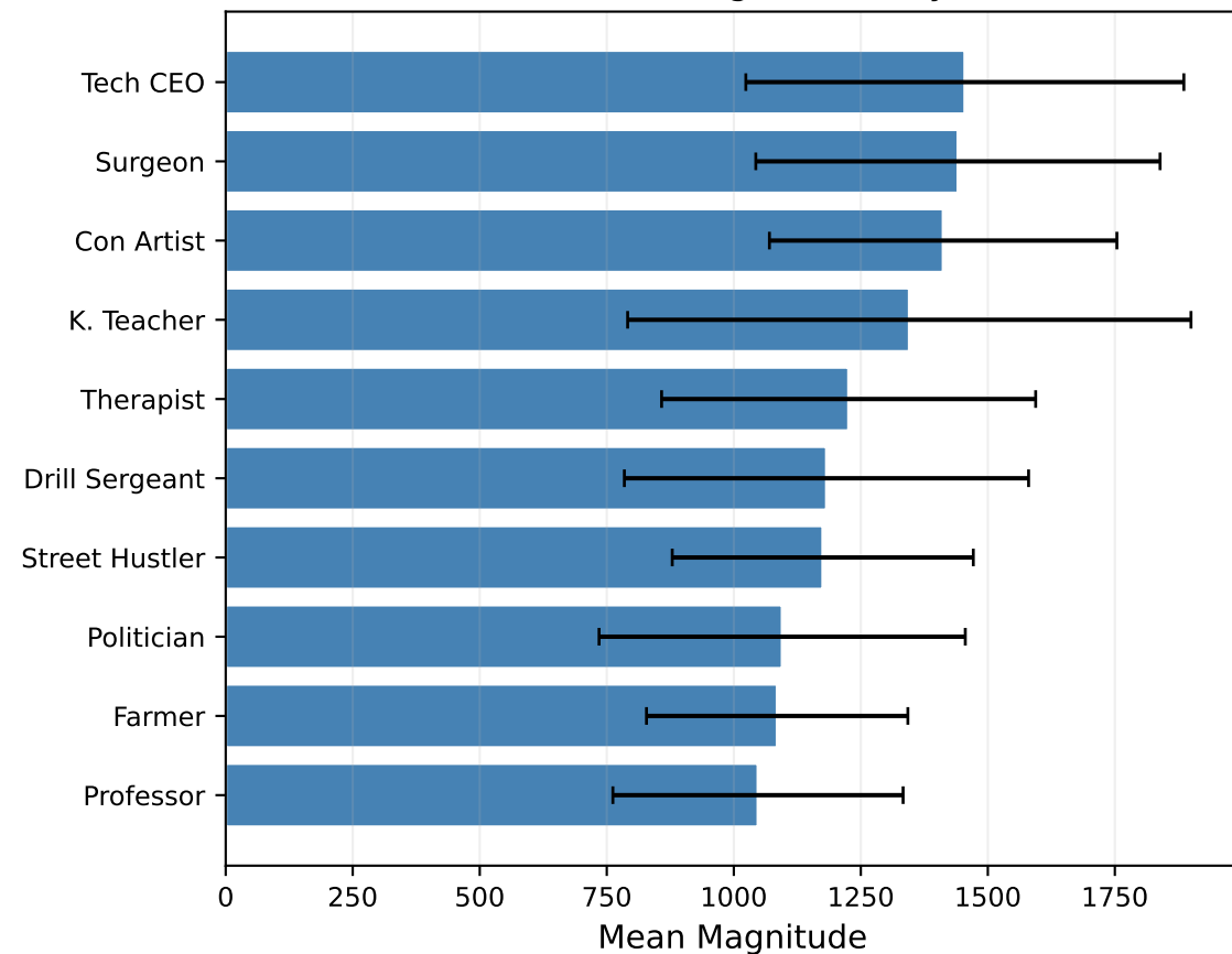
A) Per-Persona Magnitude (Layer 25)
