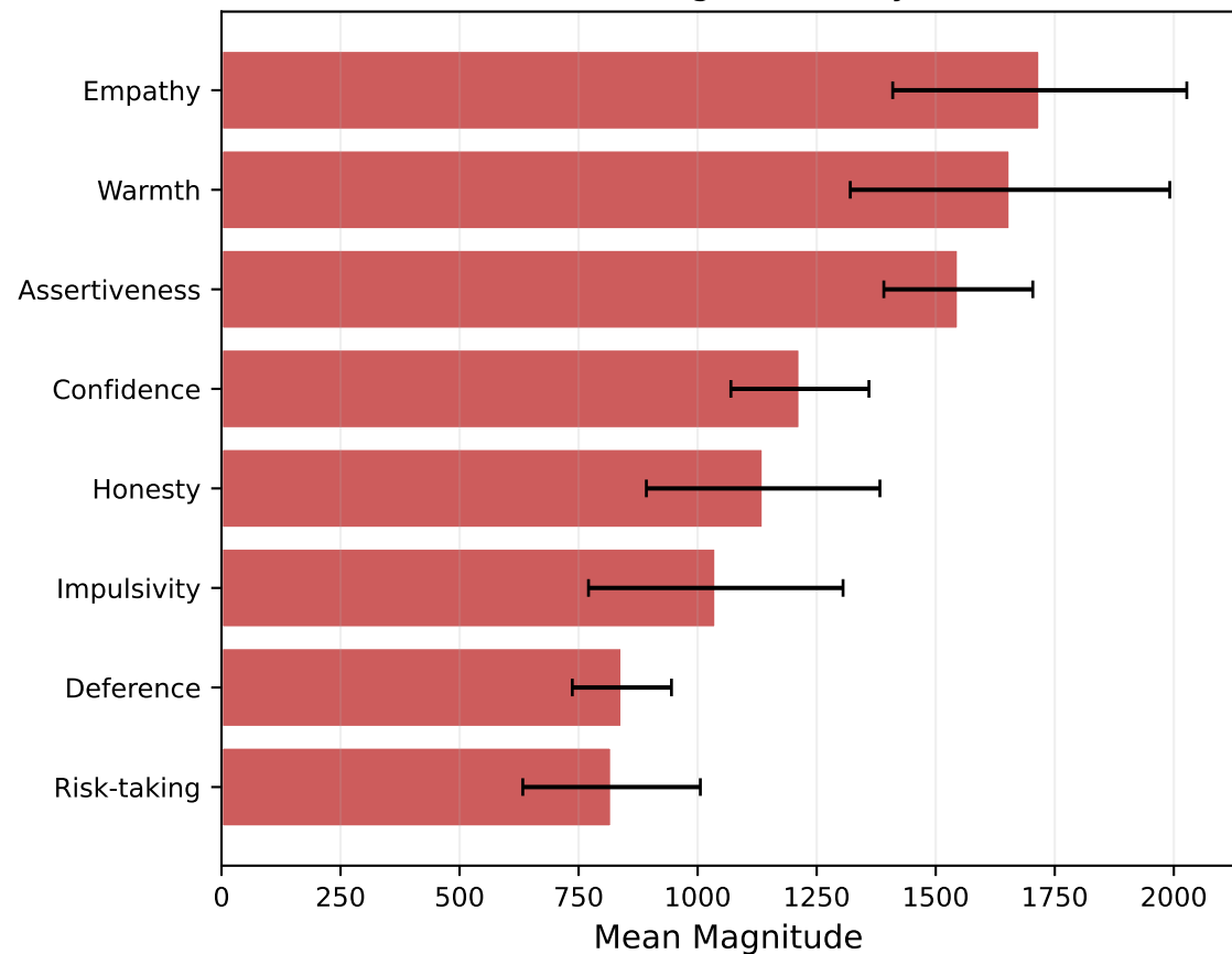
B) Per-Trait Magnitude (Layer 25)
