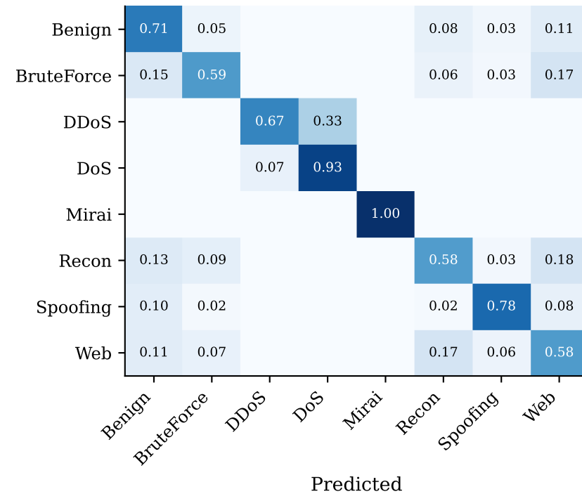
MLP
