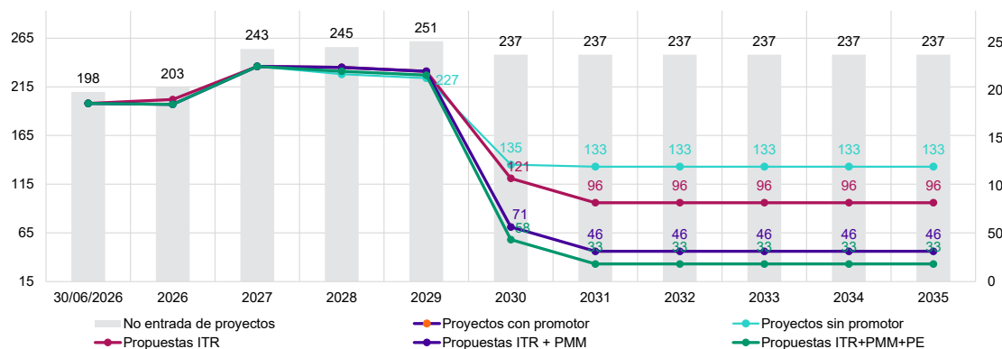
Figura 1-5 Sensibilidad de restricciones por adopción de obras y asignación de promotor
