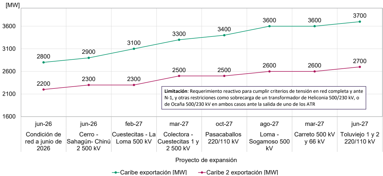
Figura 2-8 Evolución capacidad de exportación de potencia área Caribe
