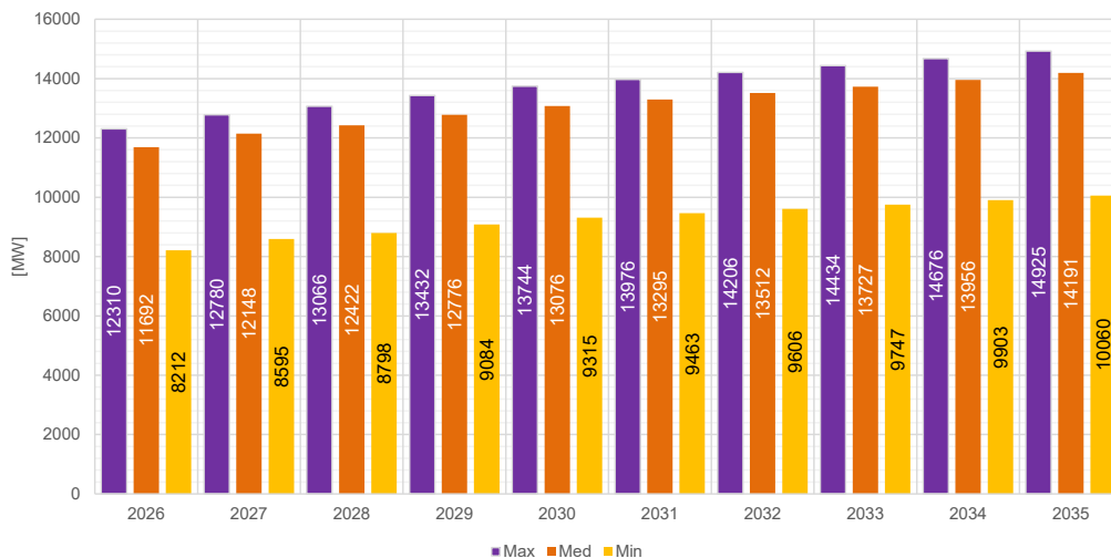
Figura 1-11 Pronóstico demanda máxima, media y mínima SIN [MW] - Años 2026 – 2035
