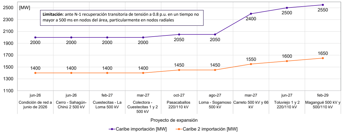
Figura 2-7 Evolución capacidad de importación de potencia área Caribe
