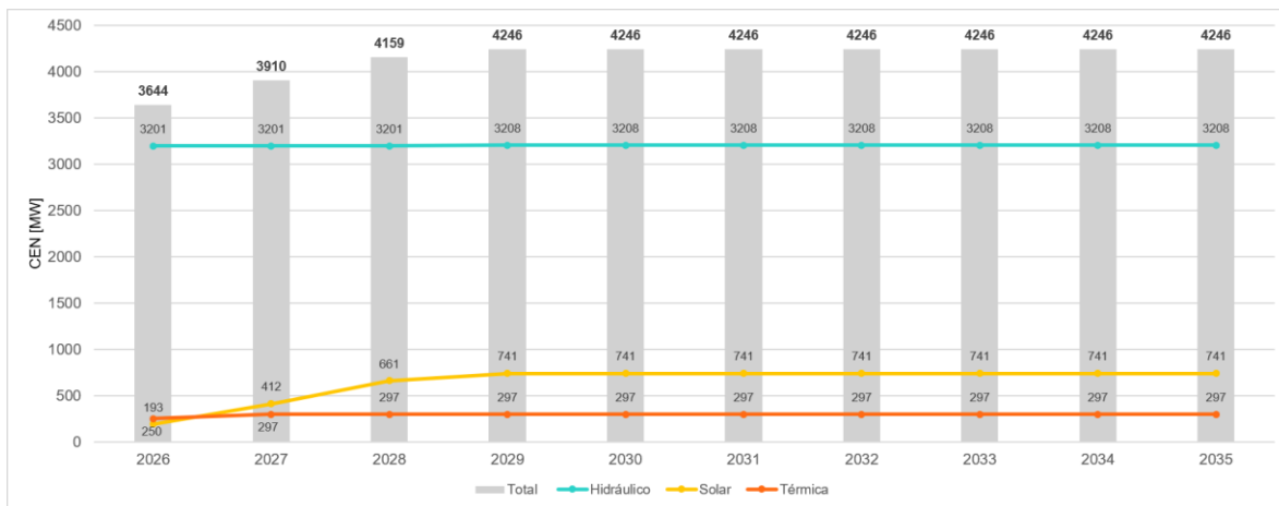
Figura 4-3 Proyección capacidad de generación en el área Oriental 2026-2035
