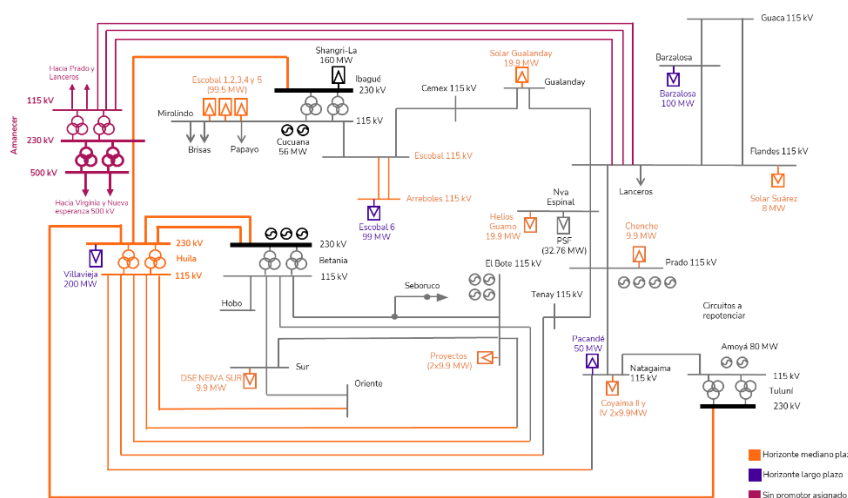
Figura 6-10 Proyectos subárea Huila – Tolima
