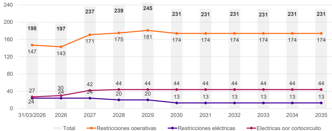
Figura 1-4 Evolución restricciones del SIN horizonte 2026 -2035
