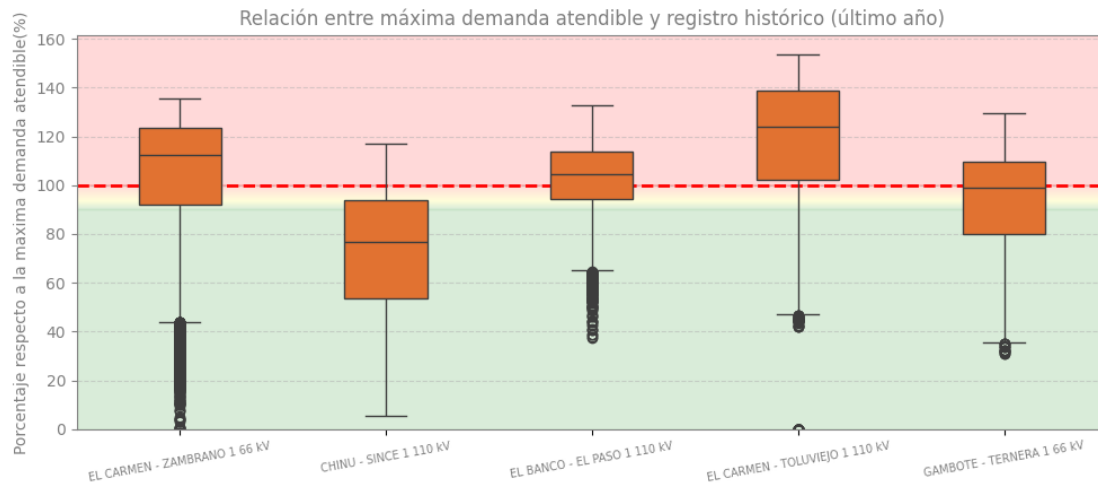
Figura 2-4 Demanda máxima atendible vs histórico Demanda
