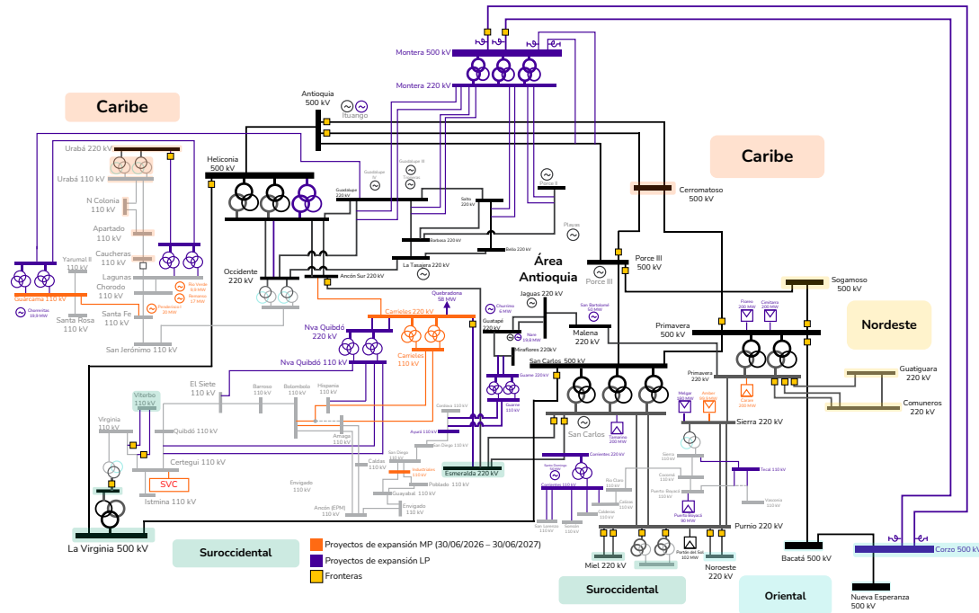
Figura 3-6. Proyectos de mayor impacto área Antioquia
