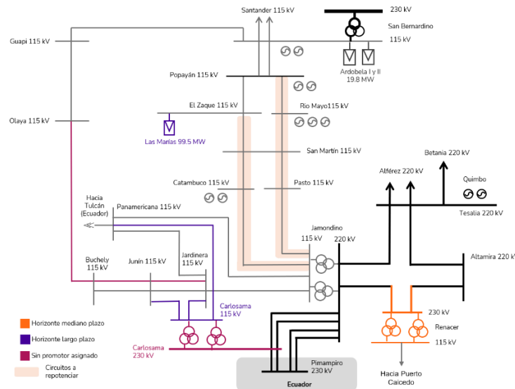
Figura 6-7 Proyectos subárea Cauca – Nariño
