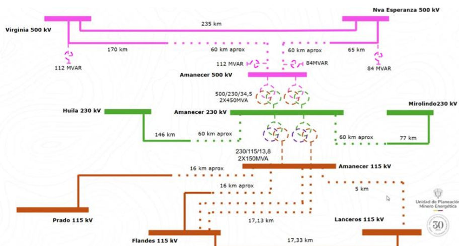
Figura 4-14. Amanecer 500/230/115 kV (tomado de Plan de Expansión de Transmisión 2024-2038 UPME)
